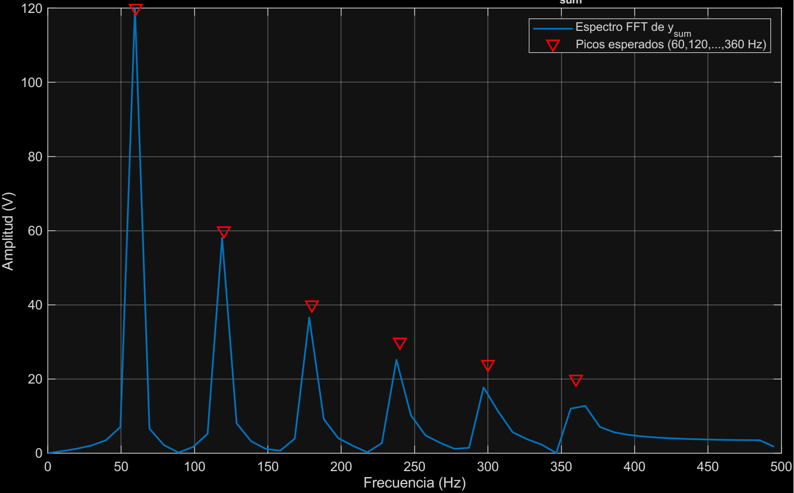
Espectro de magnitud (FFT, un solo lado) de y_{sum}
